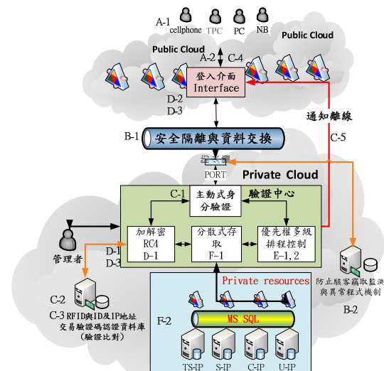
圖 3：系統架構
