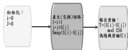
圖 13：PRGA 示意
